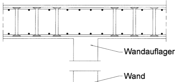
Beispiel 1: Platte
