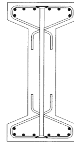
Beispiel 5: I-Träger
