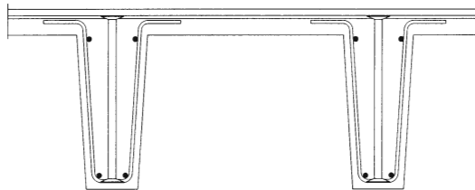
Beispiel 3: TT-Platte
