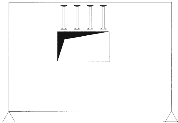
Beispiel 7: Stahlbetonwände, z.B. im Bereich von Öffnungen
