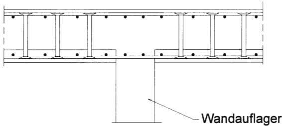
Beispiel 4: Elementdecke
