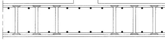
Beispiel 2: Bodenplatte
