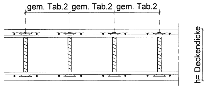
Schnitt B-B
