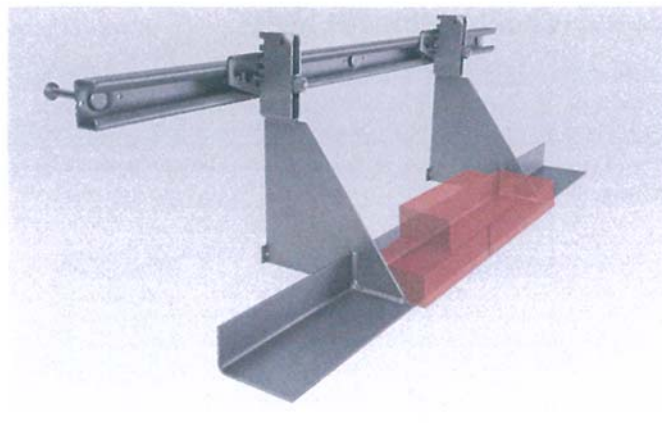
JORDAHL®-Verblenderkonsole zur Abfangung der Verblendmauerschale (Bild: Deutsche Kahneisen Gesellschaft)
